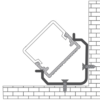
Köşe Montaj
