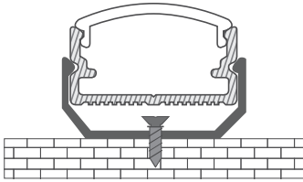
Yüzey Montaj
